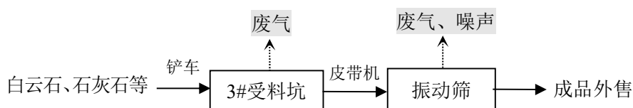
图 2-5 筛分生产线工艺流程及产排污节点图
