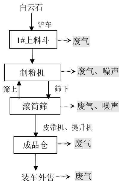
图 2-6 制粉生产线工艺流程及产排污节点图
