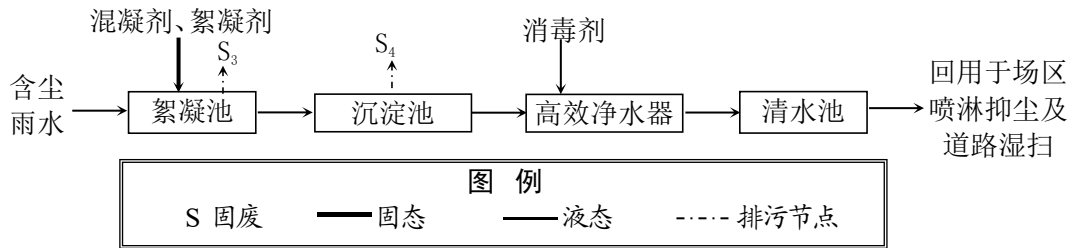
图 3 本项目含尘雨水处理工艺流程及排污节点示意图
