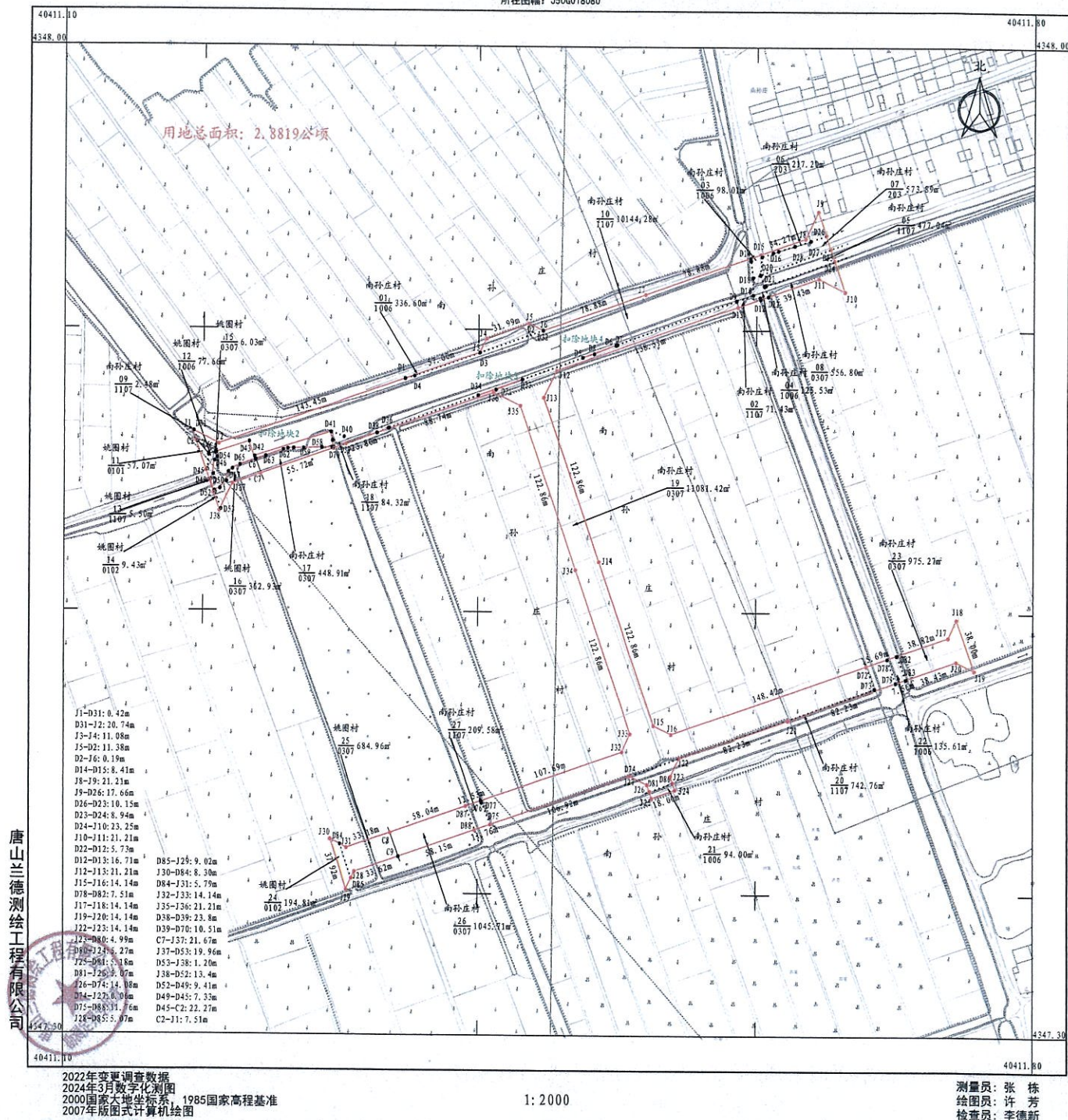
乐亭县2024年度第13批次建设用地4号地块土地勘测定界图
