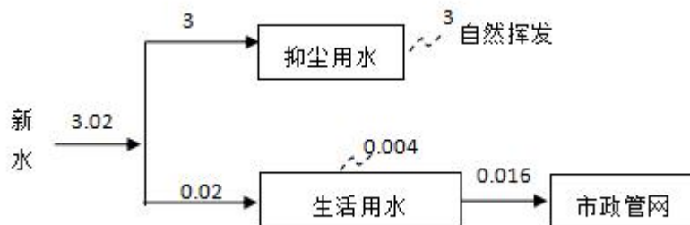
图 2-3 本项目水平衡图 m 3 /d
