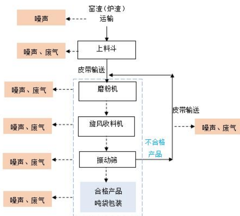
图 2-5 本项目生产工艺流程及排污节点图
