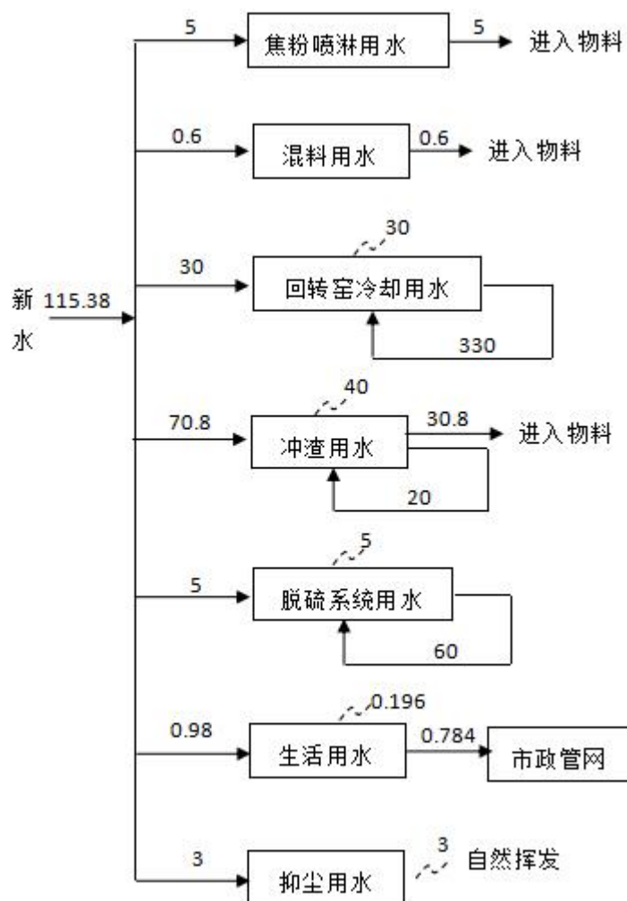
图 2-4 项目建成后全厂水平衡图 \text{m}^3/\text{d}
