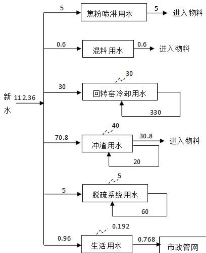
图 2-1 现有工程项目全厂水平衡图 \text{m}^3/\text{d}
