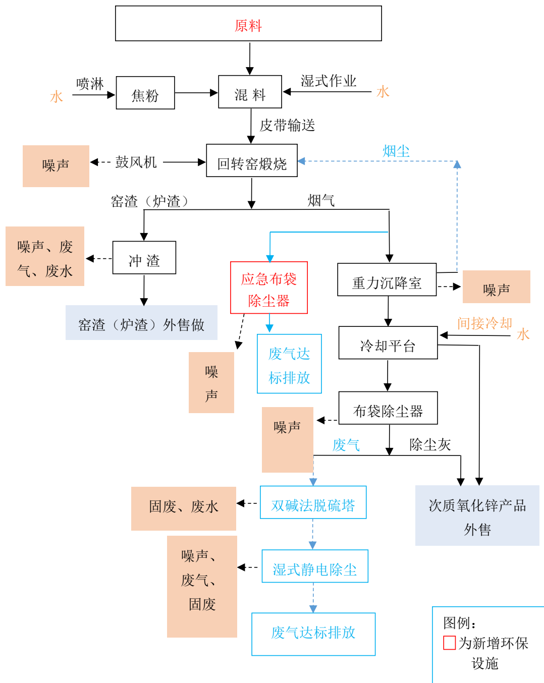
图 2-2 现有工程生产工艺流程及排污节点图
