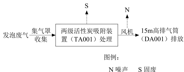
图 6 废气处理设施工艺流程及排污节点图
