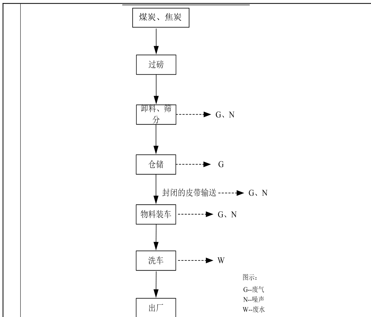
图 2-4 煤炭、焦炭仓储工艺流程及排污节点图
