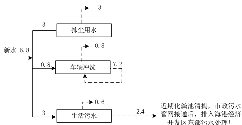
图 2-1 一期工程给排水平衡图 单位： \text{m}^3/\text{d}
