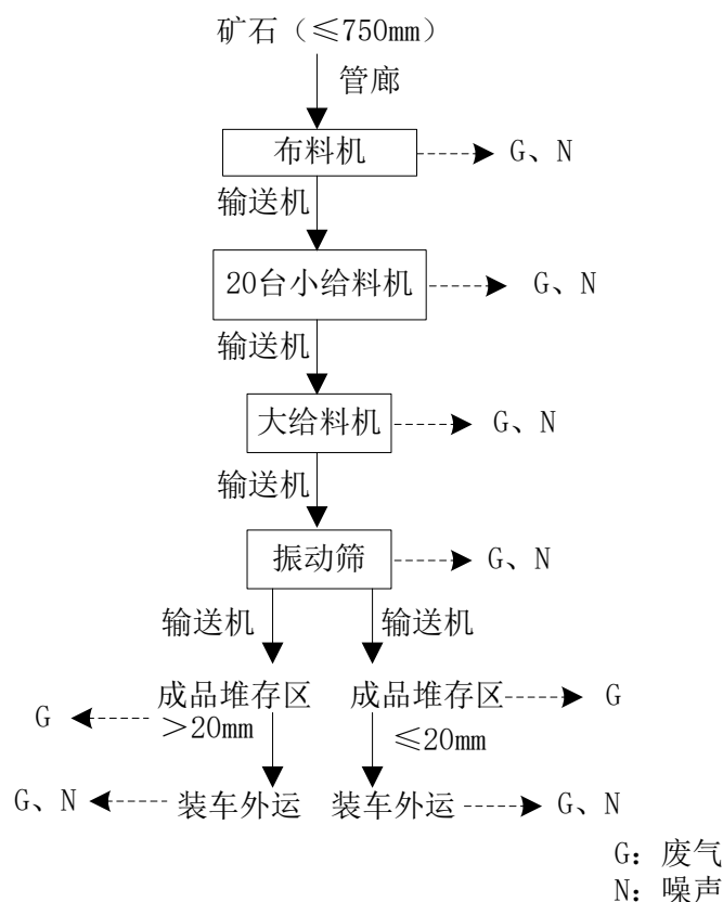
图 2-3 矿石加工生产工艺流程及排污节点图
