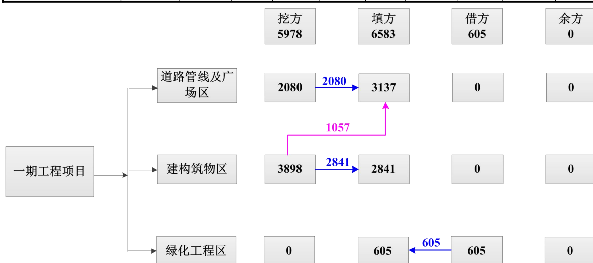
图 1-4 工程土方流向图
